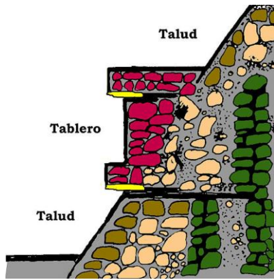
Rôzne typy systému tablero-talud:
