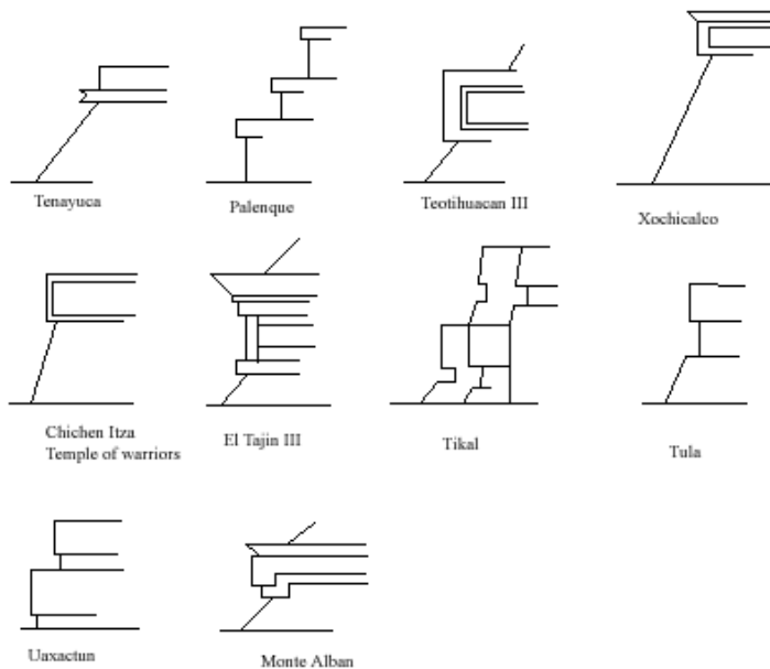
Rôzne typy systému tablero-talud:
